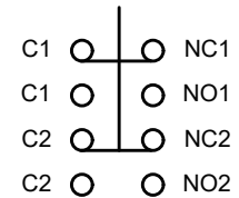
DPDT NON-ILLUM.
