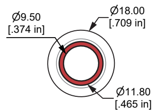
Ring-illum.
