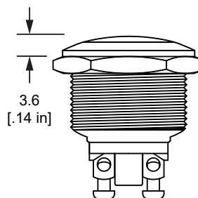
Domed Actuator
